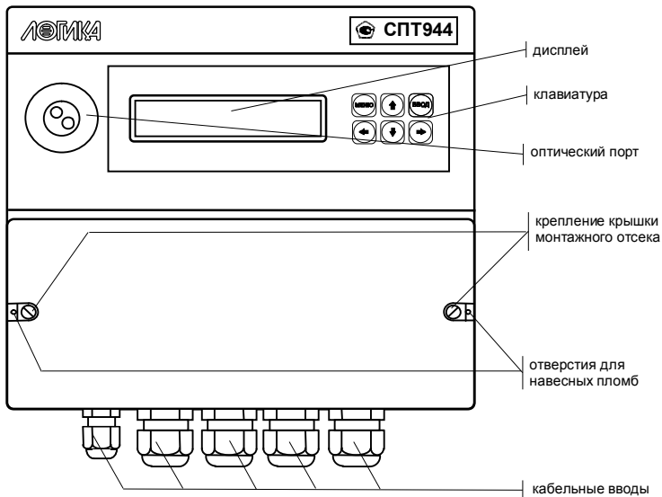
Рисунок 3.1 – Вид спереди
