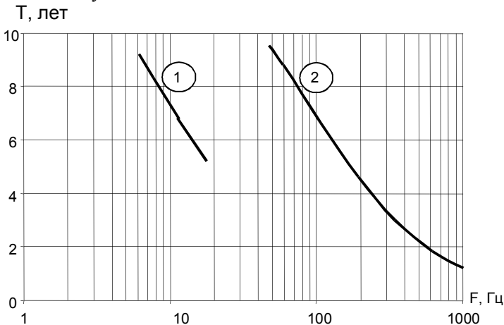
Рисунок 2.1 – Расчетный ресурс батареи (лет) при работе с низкочастотными ①, и высокочастотными ② входными сигналами.
