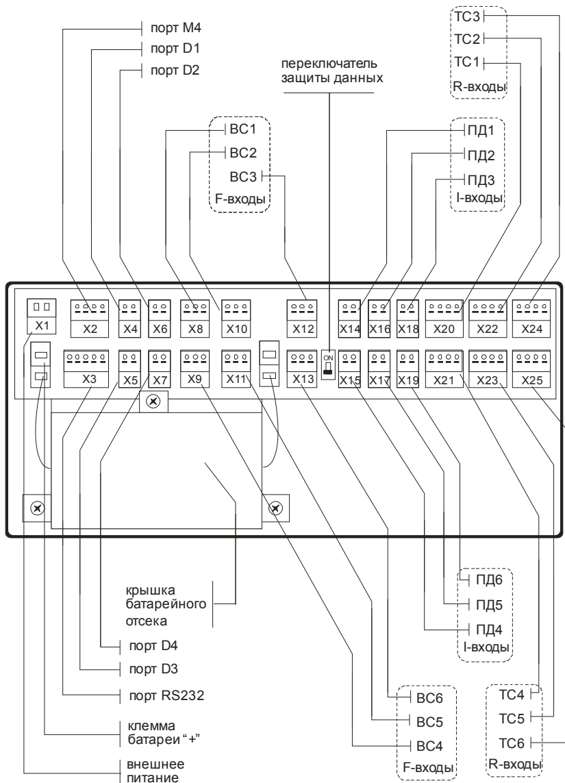
Рисунок 3.3 – Монтажный отсек
